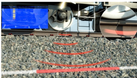
图 2: Frauscher_FTS_Railbreak. jpg
